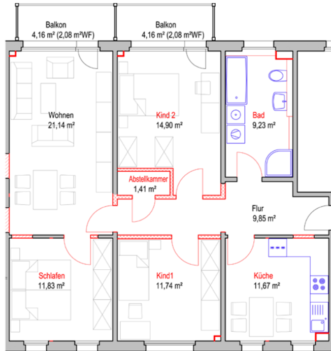
Beispiel für eine Vier-Zimmer-Wohnung, mit Rot gekennzeichnet sind die neuen Strukturen. Zeichnung: SWG
